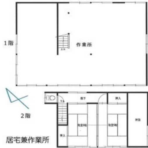
居宅兼作業所
