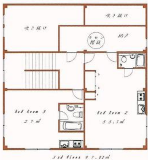
3階間取図
