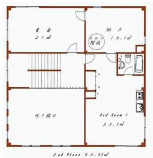
2階間取図
