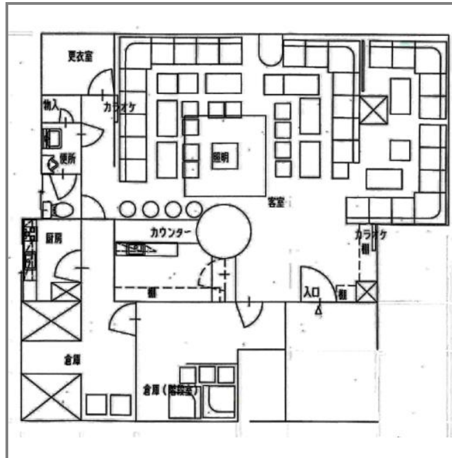
平面図
